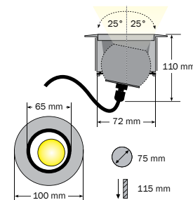
Einbautiefe mit Gehäusestecker + 60 mm Installation depth with housing plug + 60 mm Profondeur d'encastrement avec la fiche du boîtier + 60 mm
